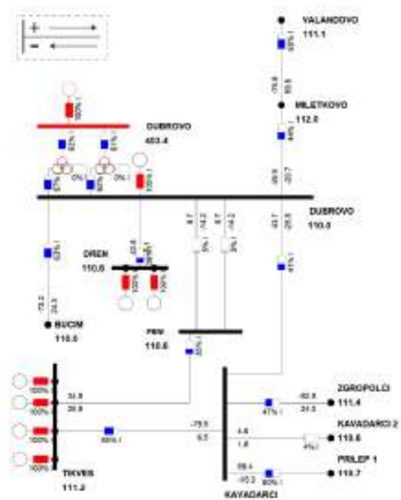
Слика 11. Напонски профил и текови на моќност за N-0, краткорочен мрежен модел, Основна Состојба
